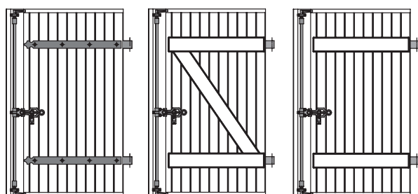
Sans barres ni écharpes
